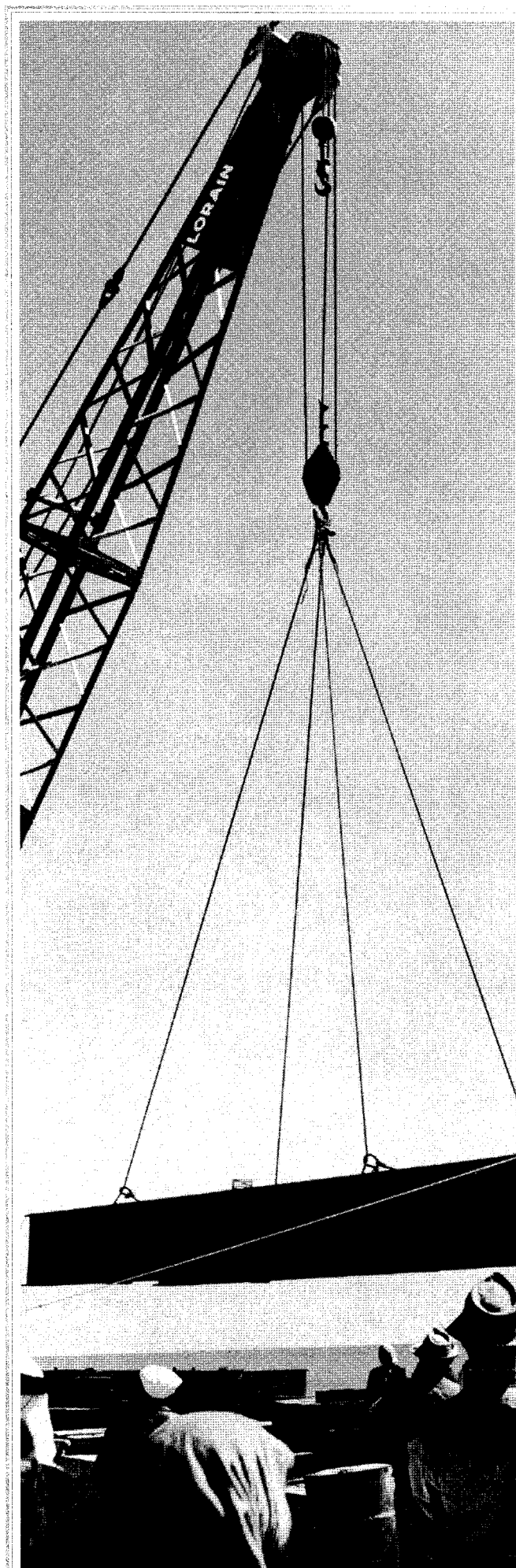
مشاهدة عملية التفريغ على رصيف الزوارق الصغيرة في الدمام Viewing offloading operation at Dammam small crafts pier.
